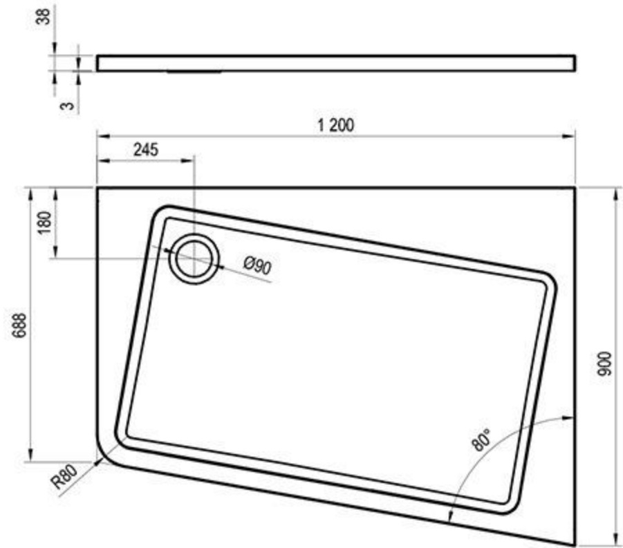
Asymetric Pro 120x90 R 10°
