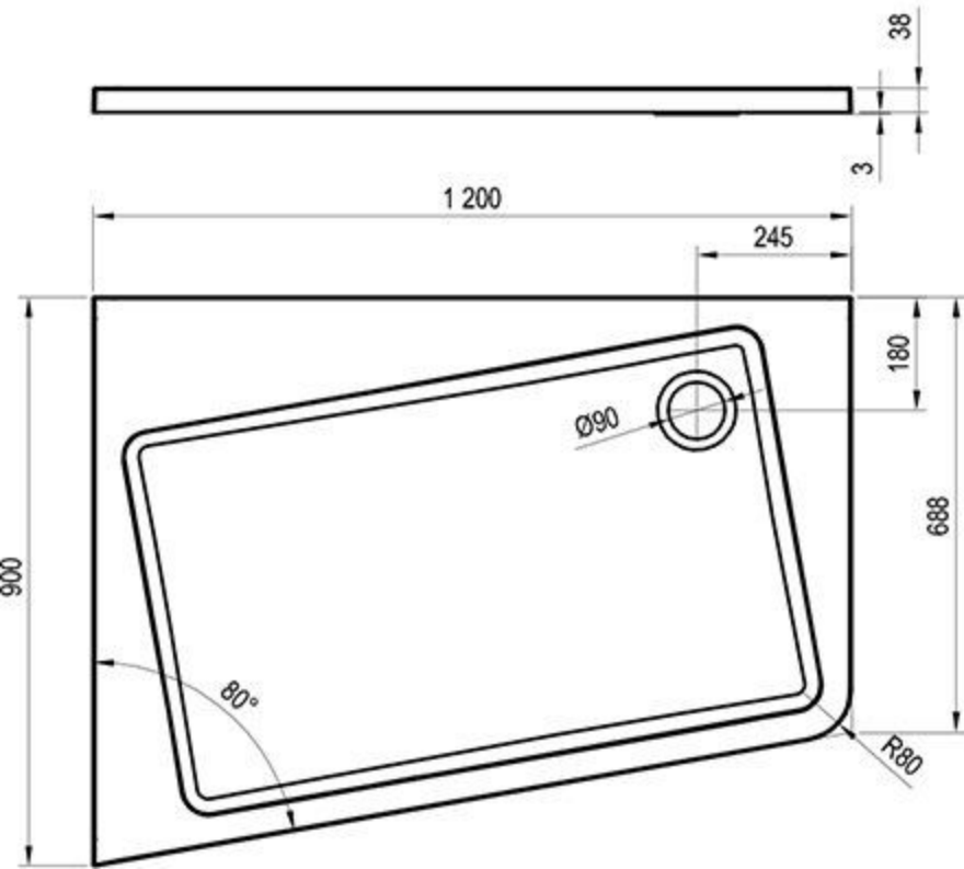
Asymetric Pro 120x90 L 10°
