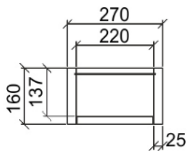
Pūdorys
