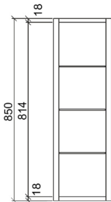
Nárys
